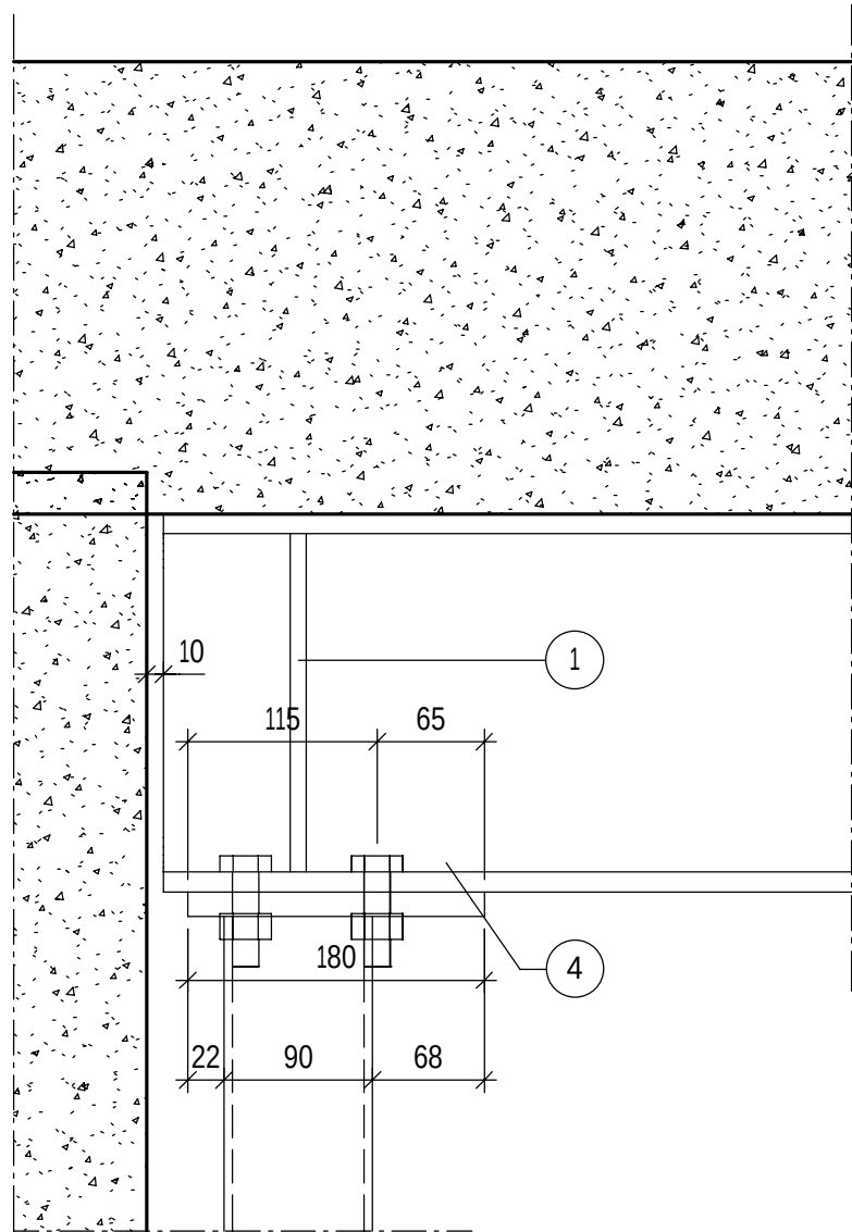
SD2 1 : 5 NYTT STÅL, LINJE C
