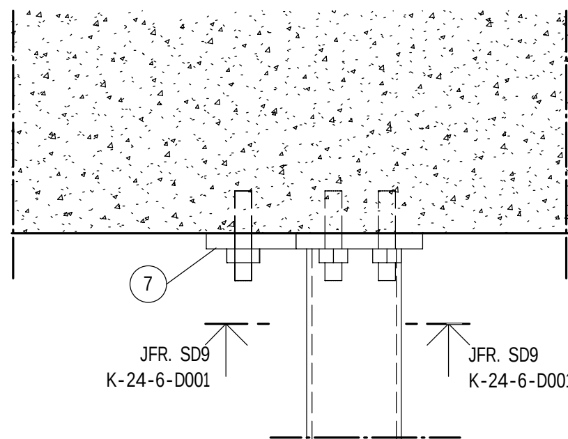
SD7 1 : 5 NYTT STÅL, HISS
