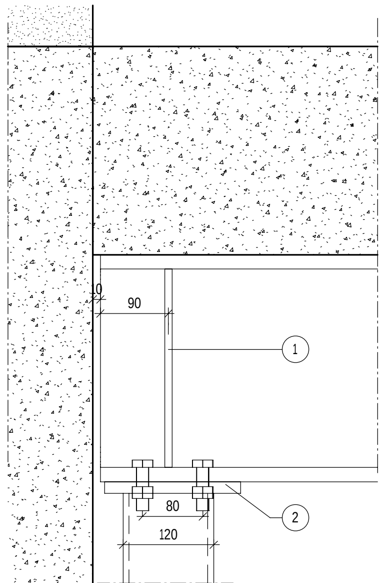
SD1 1 : 5 NYTT STÅL, LINJE C
