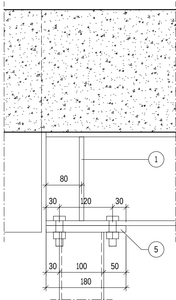
SD3 1 : 5 NYTT STÅL, TRAPPHUS
