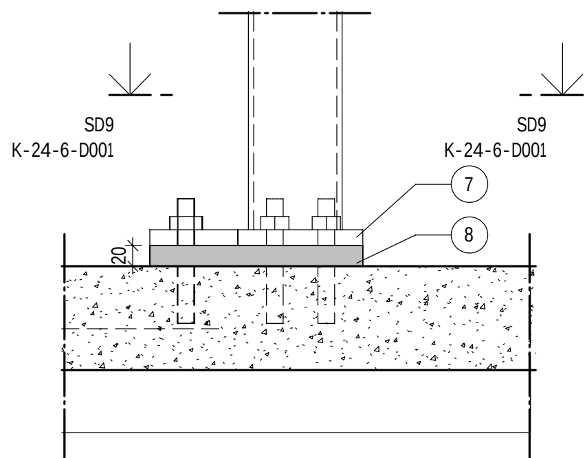
SD6 1 : 5 NYTT STÅL, HISS
