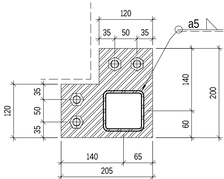
SD9 1 : 5 TOPP OCH FOTPLÅT, NYTT STÅL HISS
