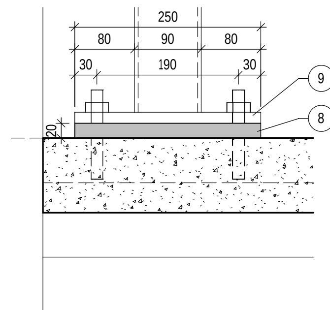
SD8 1 : 5 NYTT STÅL, HISS
