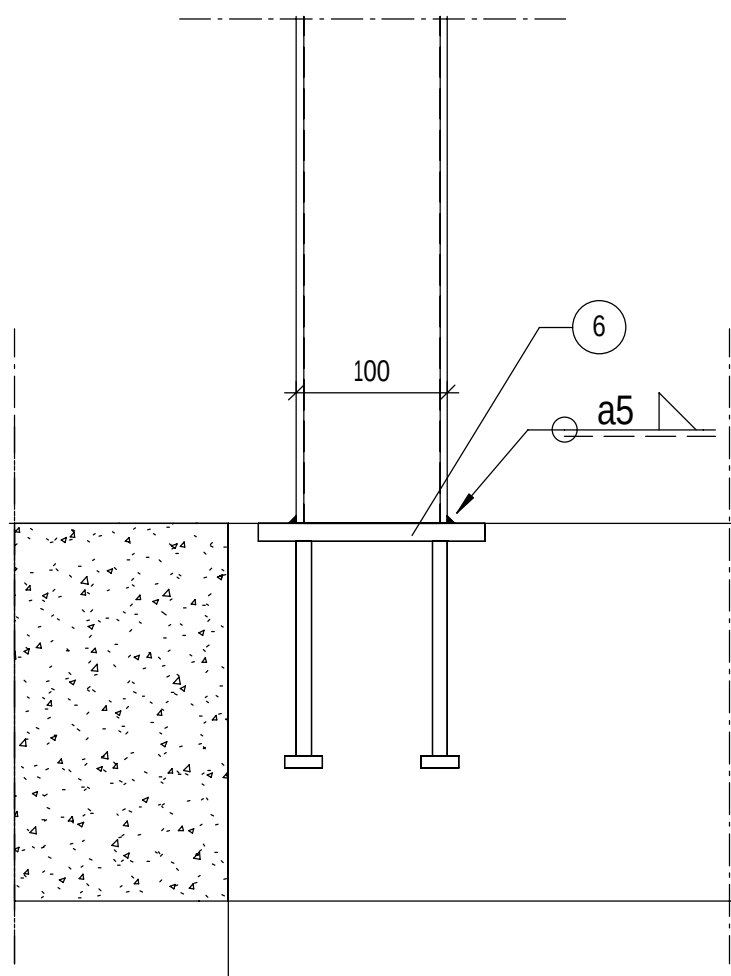
SD5 1 : 5 INGJUTNINGSGODS NYTT BJÄLKLAG TRAPPHUS
