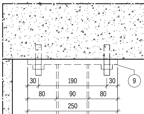
SD10 1 : 5 NYTT STÅL, HISS
